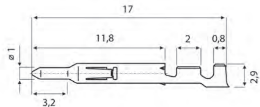
Stiftkontakt
