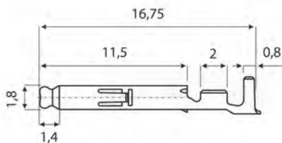
Buchsenkontakt
