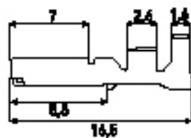
Buchsenkontakt
