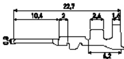
Stiftkontakt
