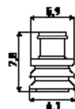
Einzeladerabdichtung / Blindstopfen
