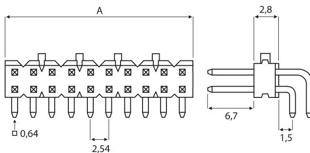
Stiftleiste gewinkelt zweireihig
