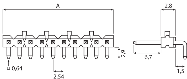
Stiftleiste gewinkelt einreihig
