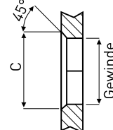
Empfohlene Montagebohrung (Gewinde, einschraubbar)
