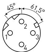
Polbild (Steckseite Gerätedose)
