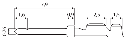
Stiftkontakt
