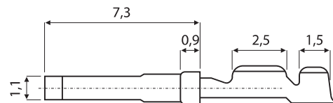
Buchsenkontakt
