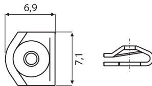
Clipverriegelung zum Aufschieben auf Steckerflansch (U-Clip mit 4-40 UNC Durchgangsloch)
