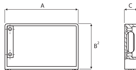
Kabelabgang seitlich
