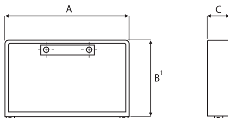
Kabelabgang gerade
