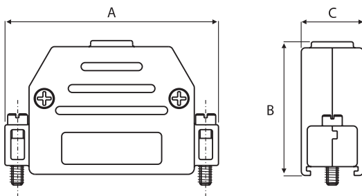
Haube mit kurzer Verriegelungsschraube
