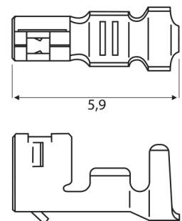
Buchsenkontakt
