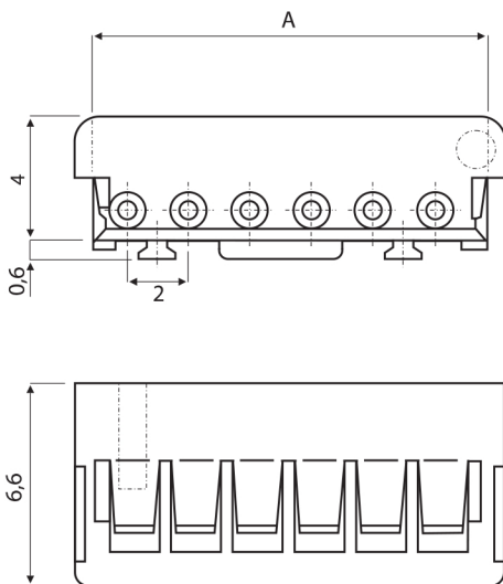
Buchsengehäuse
