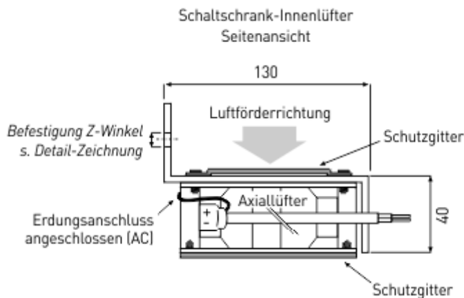
Detail Clipmontage für 35 mm Hutschiene
