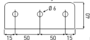
Detail Schraubmontage
