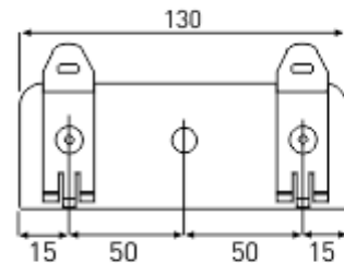
Detail Schraubmontage
