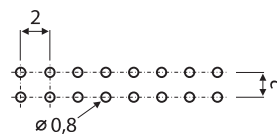
Leiterplattenlayout
