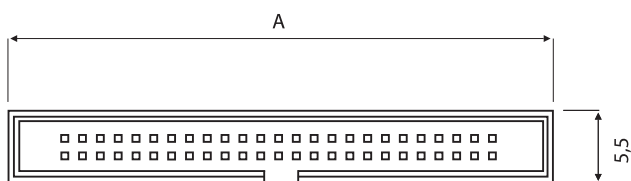
Messerleiste gerade
