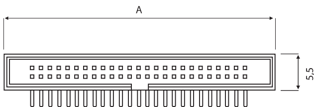
Messerleiste gewinkelt
