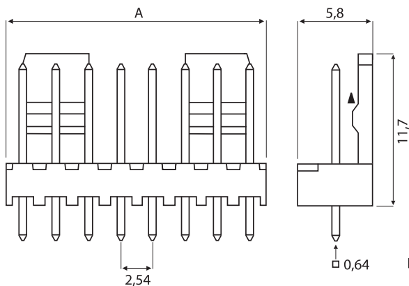
Stiftleiste gerade
