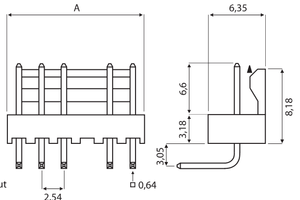
Stiftleiste gewinkelt
