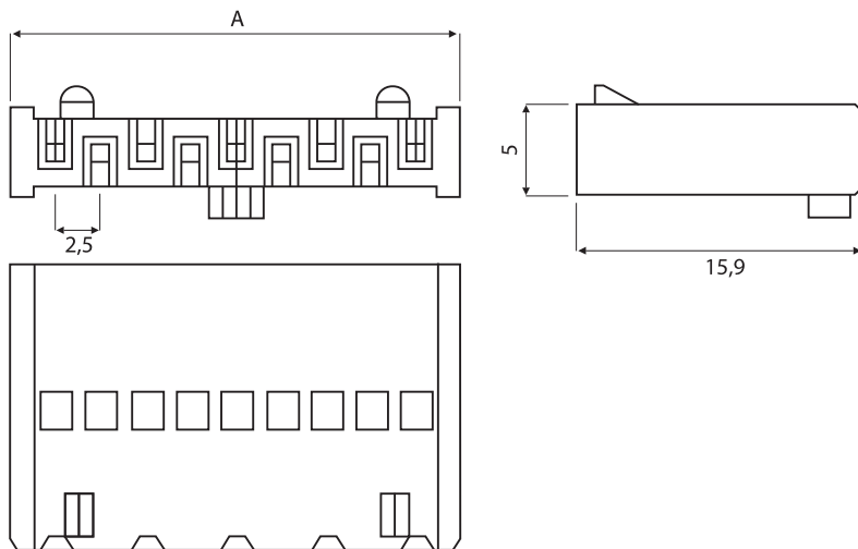
Buchsengehäuse
