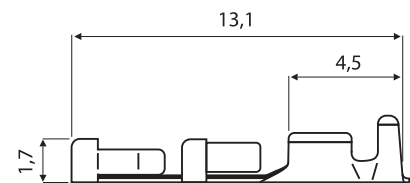
Buchsenkontakt
