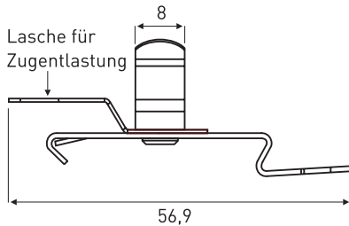
Schirmanschlussklemme mit Clip und Zugentlastung
