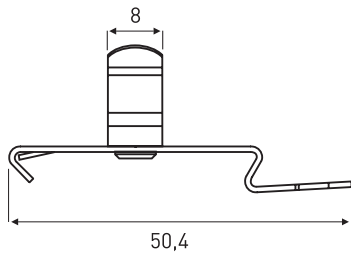
Schirmanschlussklemme mit Clip und Zugentlastung
