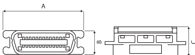
Kabelstecker
