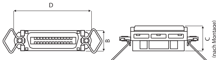
Kabeldose mit Verriegelungsklammer ohne Zugentlastung
