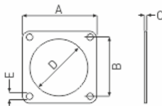
Flanschdichtung
