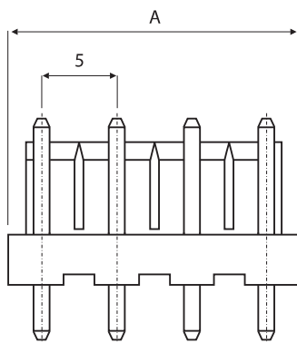
Stiftleiste gerade
