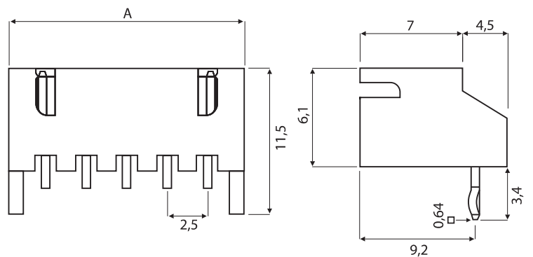
Stiftleiste gewinkelt
