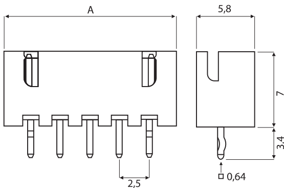
Stiftleiste gerade
