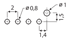
Leiterplattenlayout
