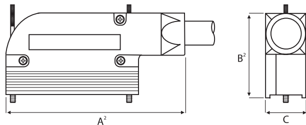
Kabelabgang seitlich
