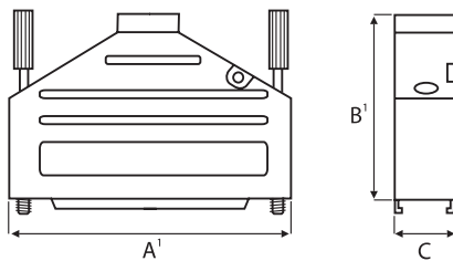
Kabelabgang gerade
