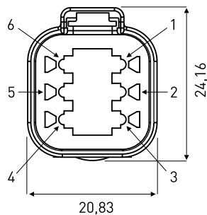
(Ansicht Steckseite)
