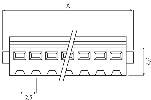
Buchsengehäuse
