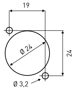
Montageausschnitt
