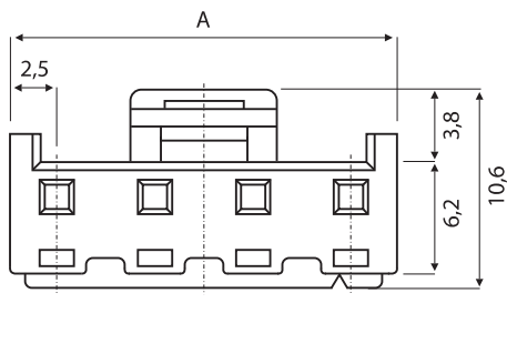
Buchsengehäuse
