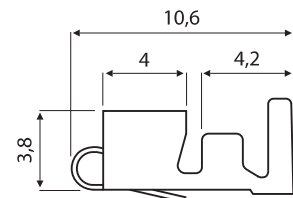
Buchsenkontakt
