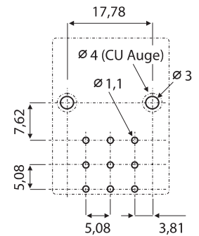
Leiterplattenlayout
