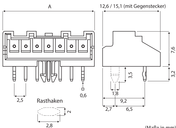
Stiftleiste gewinkelt
