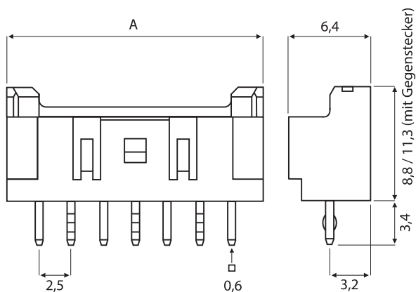
Stiftleiste gerade
