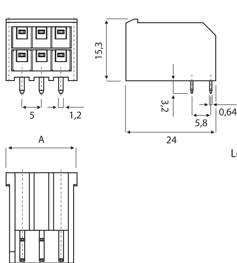
Stiftleiste gewinkelt (Typ HDS)
