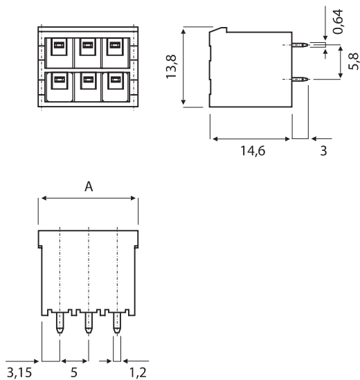
Stiftleiste gerade (Typ HDS)
