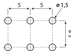
Leiterplattenlayout gewinkelt
