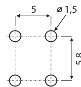
Leiterplattenlayout gerade
