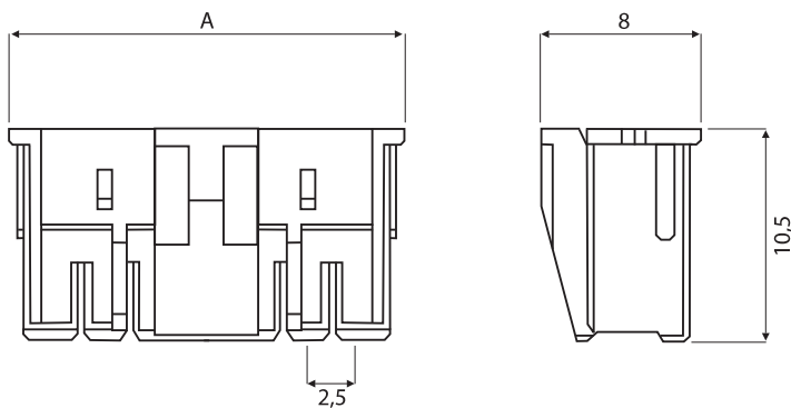
Buchsengehäuse
