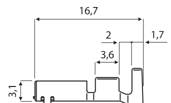
Buchsenkontakt
