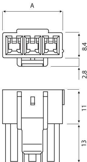
Stiftgehäuse
