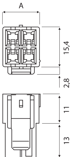
Stiftgehäuse
