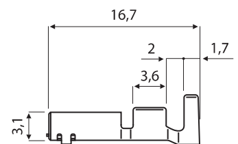
Buchsenkontakt
