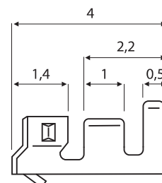
Buchsenkontakt
