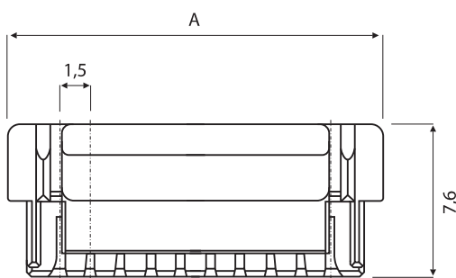
Buchsengehäuse
