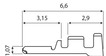
Buchsenkontakt
