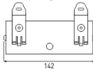
Detail Schraubmontage
