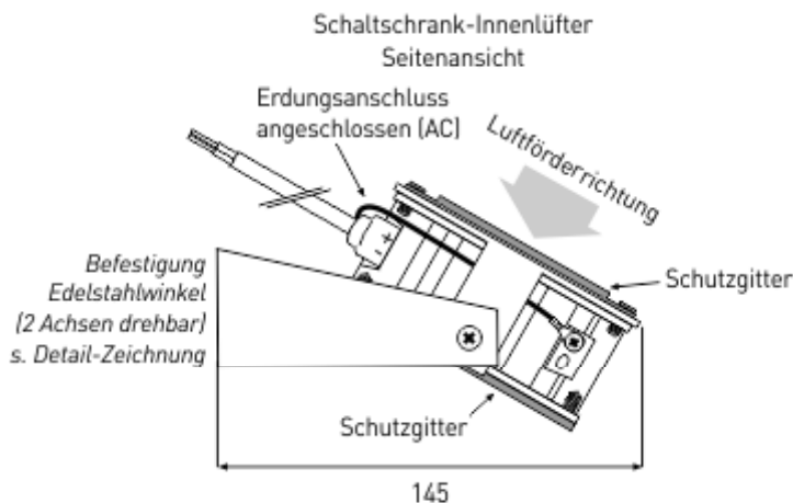
Detail Clipmontage für 35 mm Hutschiene
