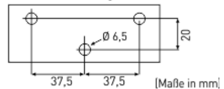
Detail Schraubmontage
