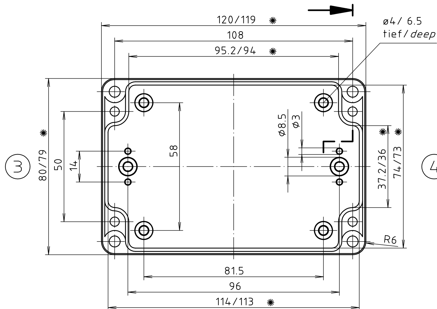
Unterteil / base
