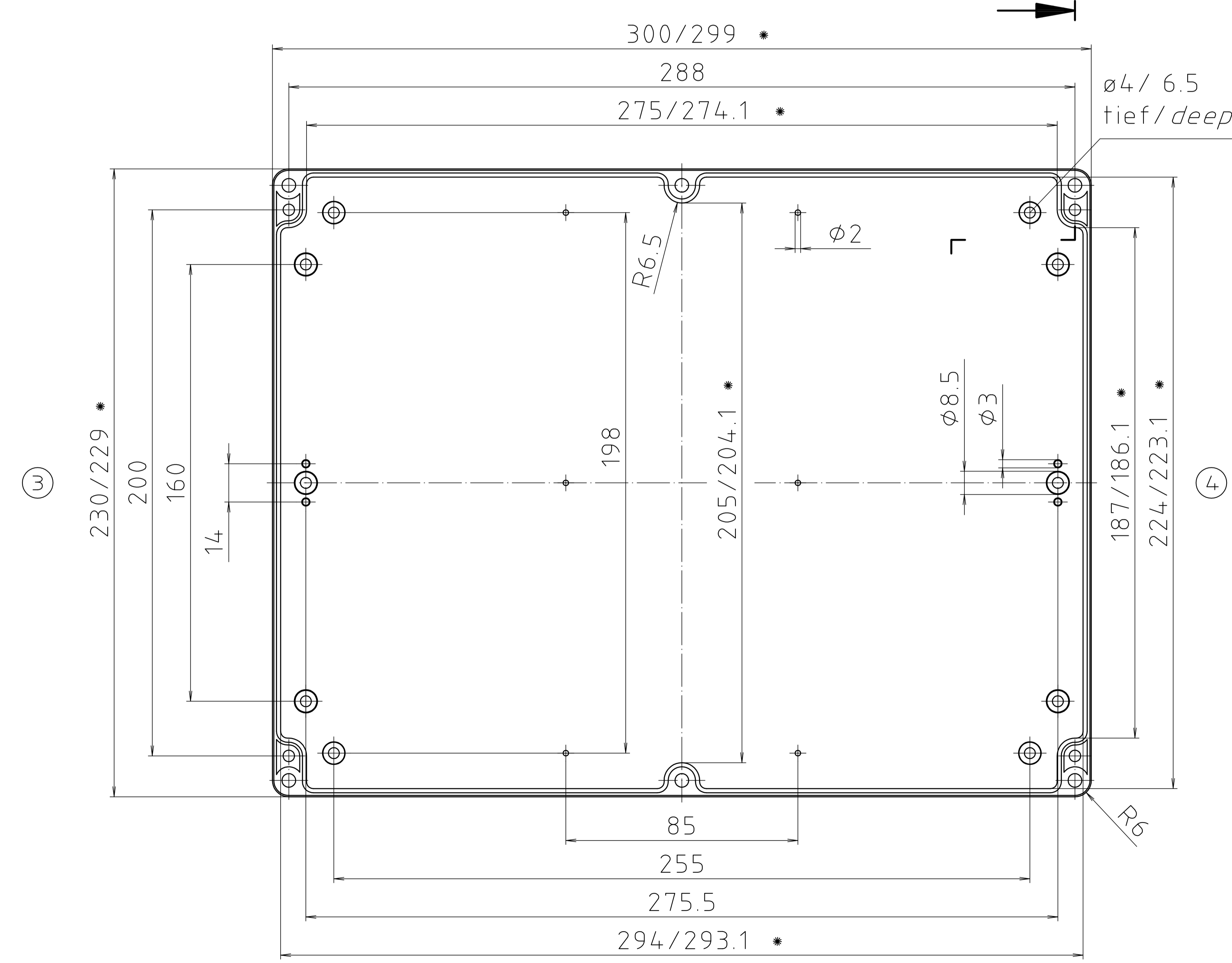
Unterteil/base
