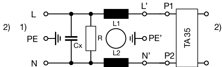
1) Line, 2) Load
