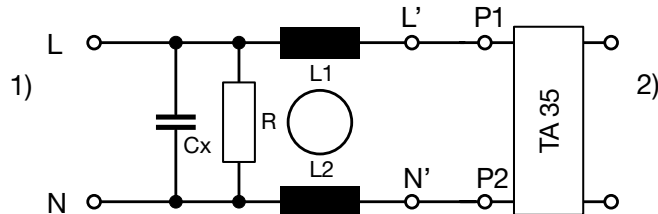
1) Line 2) Load
